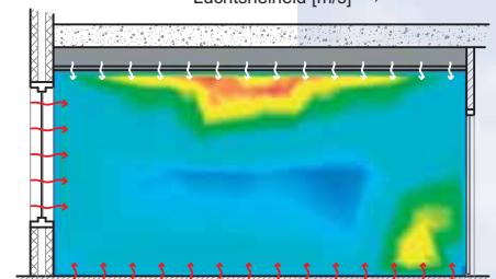
Doorsnede A_A
